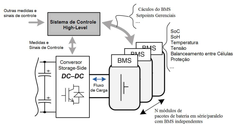
FIGURA 9 – Battery Management System (BMS). Fonte: (12)
