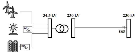
FIGURA 1 – Planta Híbrida
