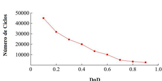
FIGURA 7 – Envelhecimento Cíclico, Fonte: (14).
