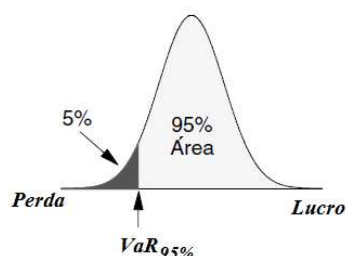
FIGURA 3 – VaR, Fonte: (3).
