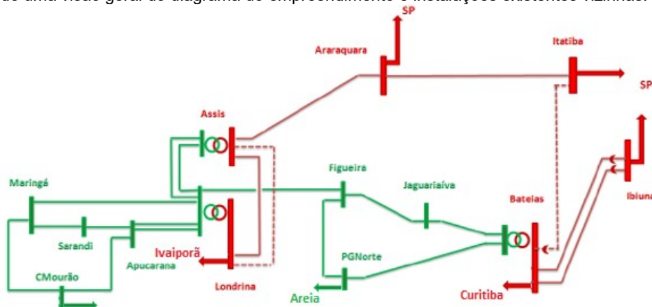
Figura 2 – Diagrama unifilar simplificado do empreendimento
