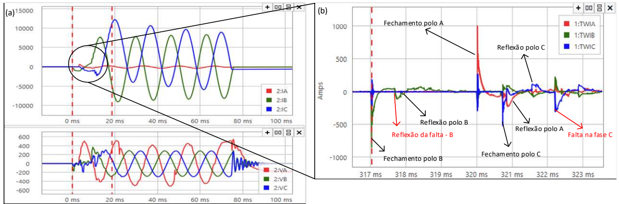
Figura 8 – Registros de 15 kHz (a) e 1.5 MHz (b) do religamento manual
