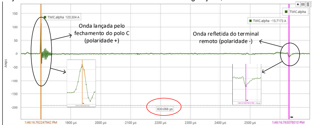
Figura 4 – Medição da diferença de tempo das ondas lançada e refletida do terminal remoto para a fase C
