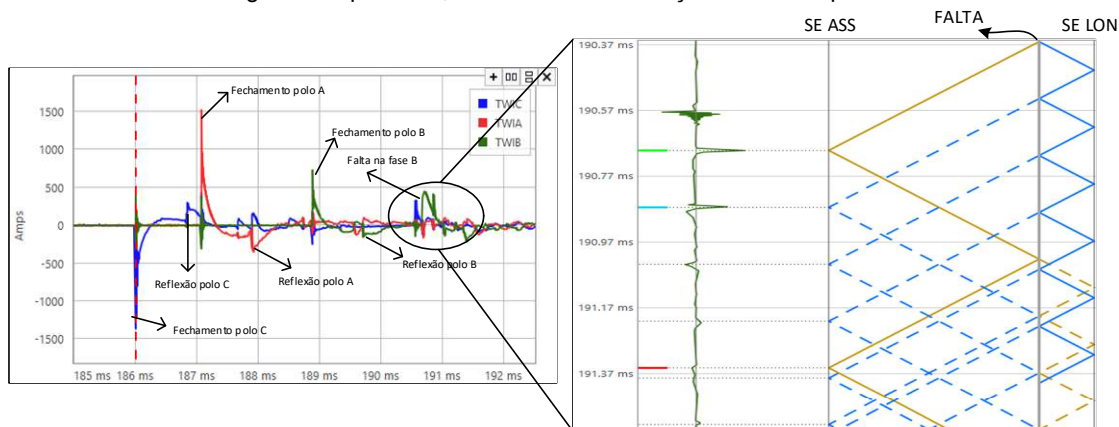
Figura 7 – Diagrama de Bewley com destaque no momento da reincidência da falta na fase B
