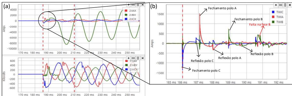
Figura 6 – Registros de 8 kHz (a) e 1.5 MHz do religamento automático (b)
