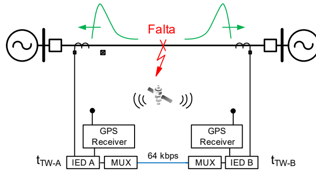
Figura 1 – Implementação do DETWFL em IED de proteção diferencial de linhas
