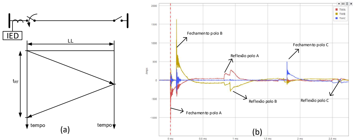
Figura 3 – Representação do teste de energização (a) Registro de 1.5 MHz do teste de energização (b)
