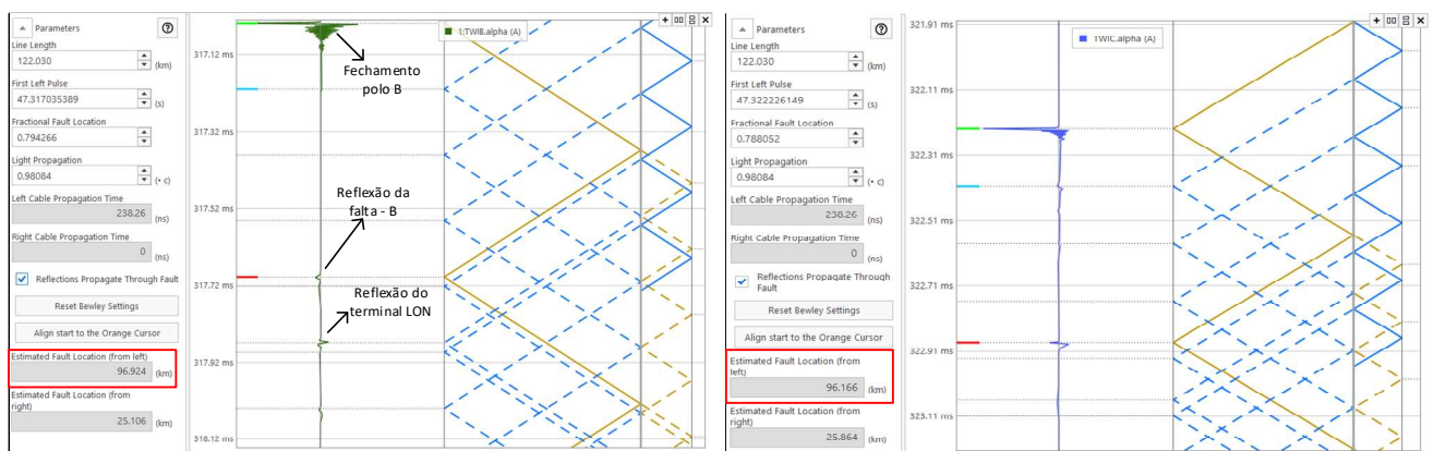
Figura 9 – Diagrama de Bewley religamento sob falta BG (a) e envolvimento da fase C na falta (b)
