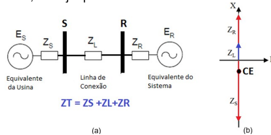
FIGURA 1 - Sistema Equivalente de Duas Barras
