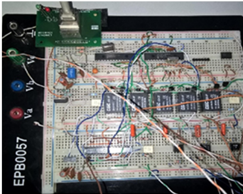
Fig. 3 – Protótipo do Módulo de Comando.
